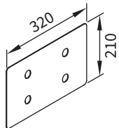
Abdeckblech für Distanzplatte und Distanzhalter bei Isolierputz 320 × 210 × 2 mm
