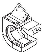
Dachsparrenhalter 150 mm, 5°–35° Lasche 150 mm
