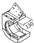
Dachsparrenhalter 150 mm, 5°–35° Lasche 150 mm
