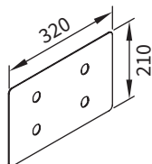
Abdeckblech für Distanzplatte und Distanzhalter bei Isolierputz 320 × 210 × 2 mm
