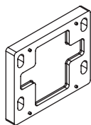
Distanzplatte Wand 180 × 150 × 20 mm; schwarz
