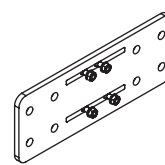
Befestigungsplatte A 430 × 160 × 12 mm
