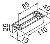
Halteraufnahme für Sparren mit 14 mm Breite für Montage direkt auf Wintergartensparren
