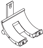
Koppelhalter Kassette mittig Neigungseinstellung 5°–45°
