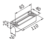
Halteraufnahme für Sparren mit 25 mm Breite für Montage direkt auf Wintergartensparren
