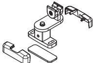
Schienenhalter oben beweglich 100 mm
