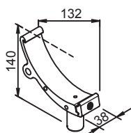
Kassetten- / Gehäuse- abstützung auf Rahmen 140 mm
