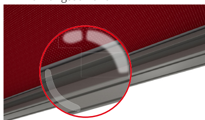
2 tracfix Tuchführung – ohne Spalt zur Führungsschiene 1)
