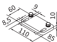
Adapterplatte für Schienenhalter 110 × 60 × 10 mm
