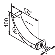
Kassetten- / Gehäuse- abstützung auf Rahmen 100 mm
