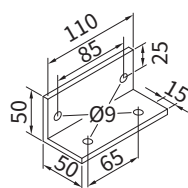
Befestigungswinkel
