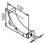
Kassetten- / Gehäuse- abstützung auf Rahmen 100 mm
