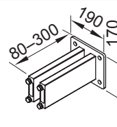
Distanzhalter für Wandhalter 70617. und 70600.
