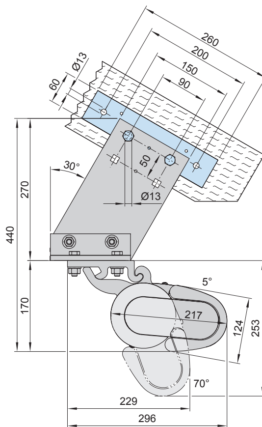
Dachsparrenhalter mit Zusatzlasche für 71659.
