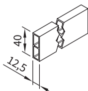
Distanzleiste für Wandanschluss Meterware
